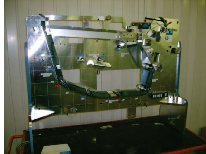
Door Panel CF
